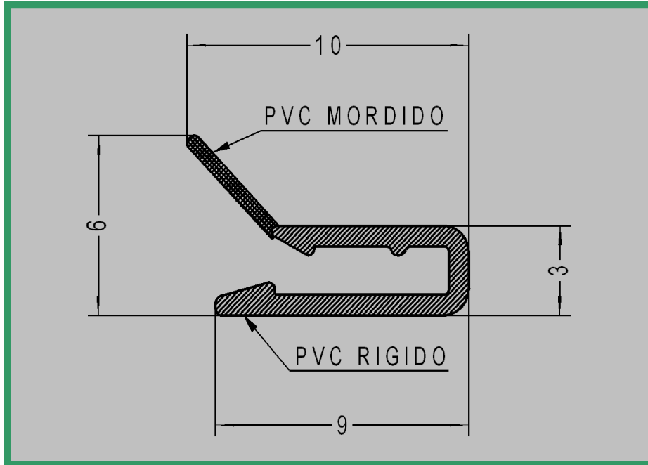
Profilo 3010.16 Materiale : PVC COESTRUSO
