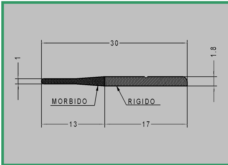
Profilo 3010.14 Materiale : PVC COESTRUSO
