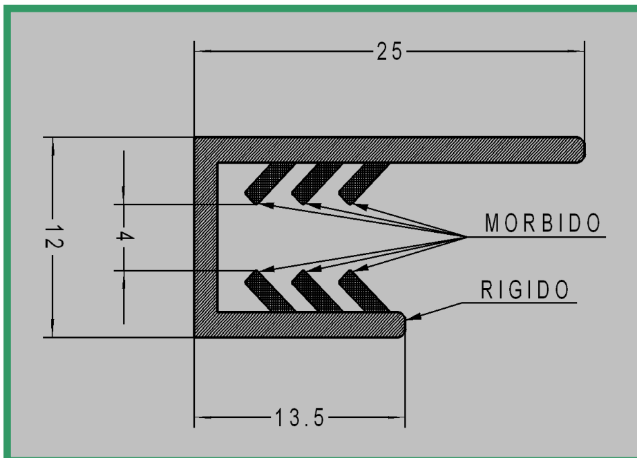
Profilo 3010.12 Materiale : PVC COESTRUSO
