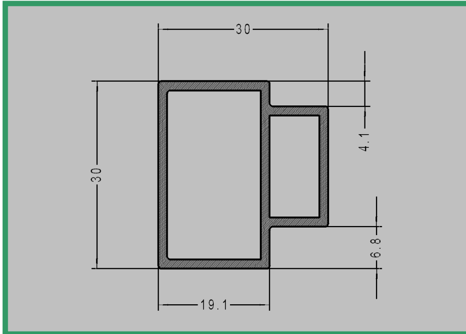
Profilo 3010.04 Materiale : ABS
