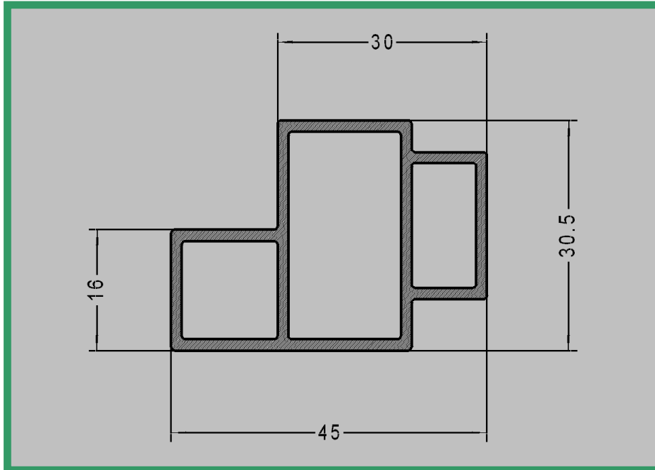
Profilo 3010.02 Materiale : ABS
