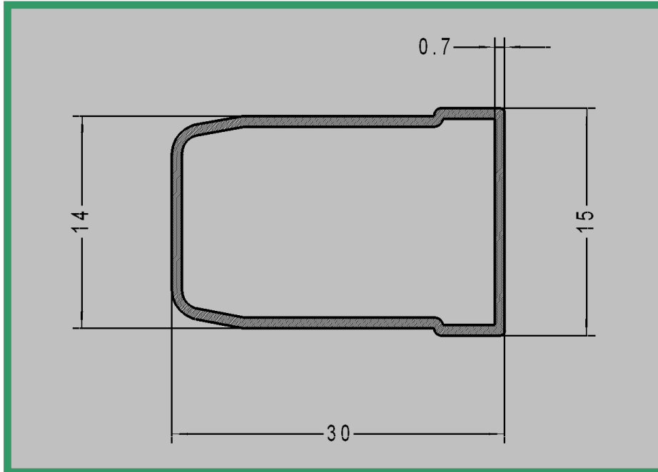
Profilo 3010.05 Materiale : ABS
